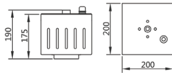
1/2" NPT Conduit Mount
