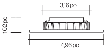
Boîte de jonction
