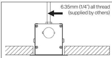
Drywall Flange
